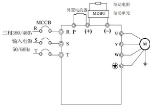
图 3.5 三相 132-315kW
