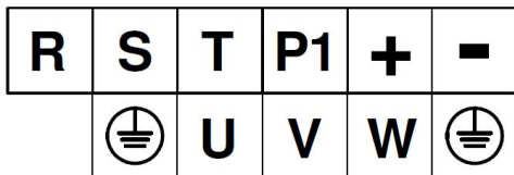
图 3-17 200kW-315kW 主回路接线端子
