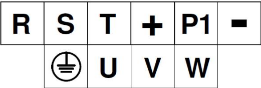
图 3-17 132kW-160kW（5063 型）主回路接线端子
