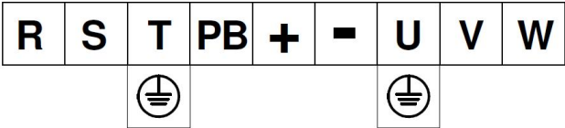
图 3-16 75kW-110kW（5061B 型）主回路接线端子
