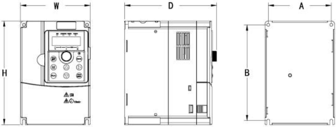
图 6-1 JAC300 系列 塑胶结构外型尺寸及安装尺寸示意图
