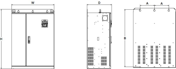
图 6-2 JAC300 系列 钣金结构外型尺寸及安装尺寸示意图
