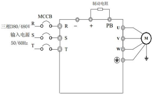
图 3.3 三相 0.75-37kW 接线标准
