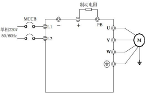
图 3-2 单相 0.75-2.2kW 接线标准
