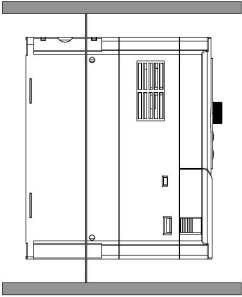
法兰式安装
