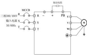
图 3.4 三相 45-110kW 接线标准（制动电阻选配）
