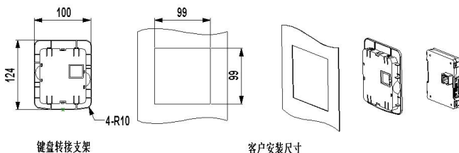
图 6-4 键盘支架开口尺寸
