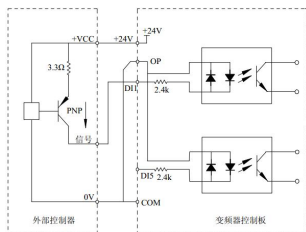
图 3-28 源型接线方式
