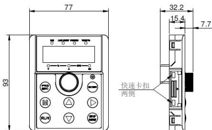
图 6-3 键盘的外型尺寸
