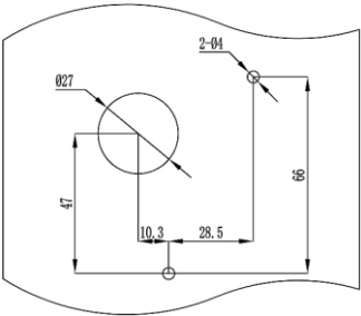
45-450KW 键盘螺丝固定开口尺寸
