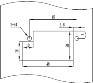
(0.75-37KW) 键盘螺丝固定开口尺寸
