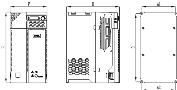
图 6-1 HC100 系列 塑胶结构外型尺寸及安装尺寸示意图
