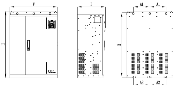
图 6-2 HC100 系列 钣金结构外型尺寸及安装尺寸示意图
