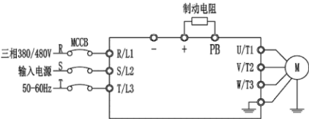
图 3.3 三相 0.75-37kW 接线标准 三相 45-110kW 接线标准（制动电阻选配）
