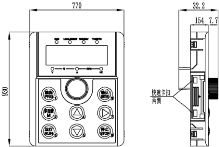
45-450KW 键盘外型尺寸
