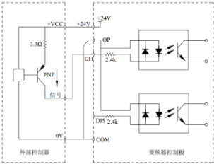
图 3-28 源型接线方式
