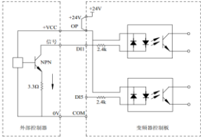
图 3-26 漏型接线方式
