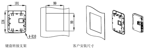
图 6-4 键盘支架开口尺寸
