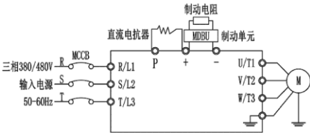
图 3.5 三相 132-315KW
