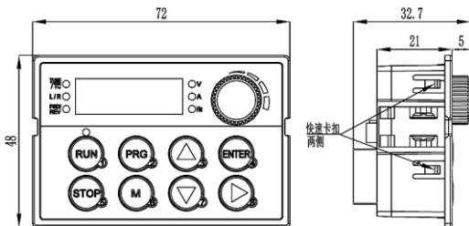
(0.75-37KW) 键盘外型尺寸
