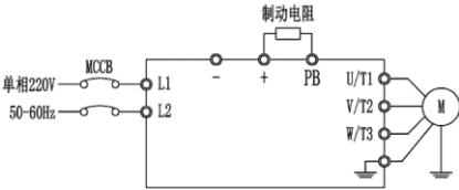
图 3-2 单相 0.75-2.2kW 接线标准
